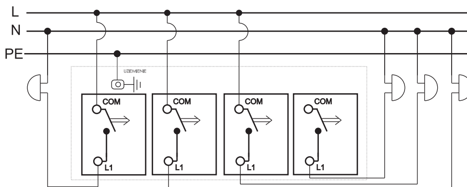
Schemat podłączenia łącznika zwiernego poczwórnego.
